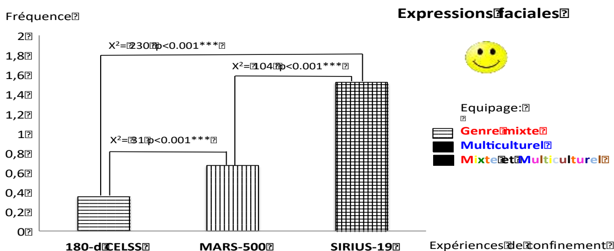
Figure 2. Occurrence des expressions faciales en fonction des qualités intrinsèques d'équipages confinés simulant des voyages interplanétaires. Le test du Chi2 est calculé sur les valeurs absolues.
